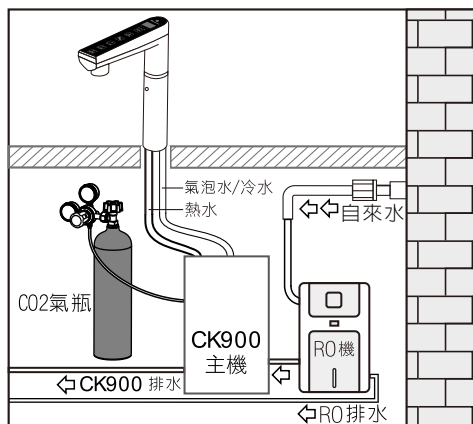
安裝說明圖
