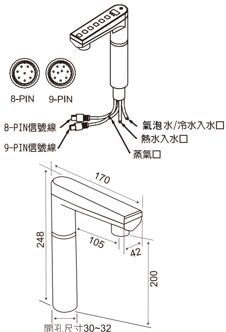
安裝說明圖
