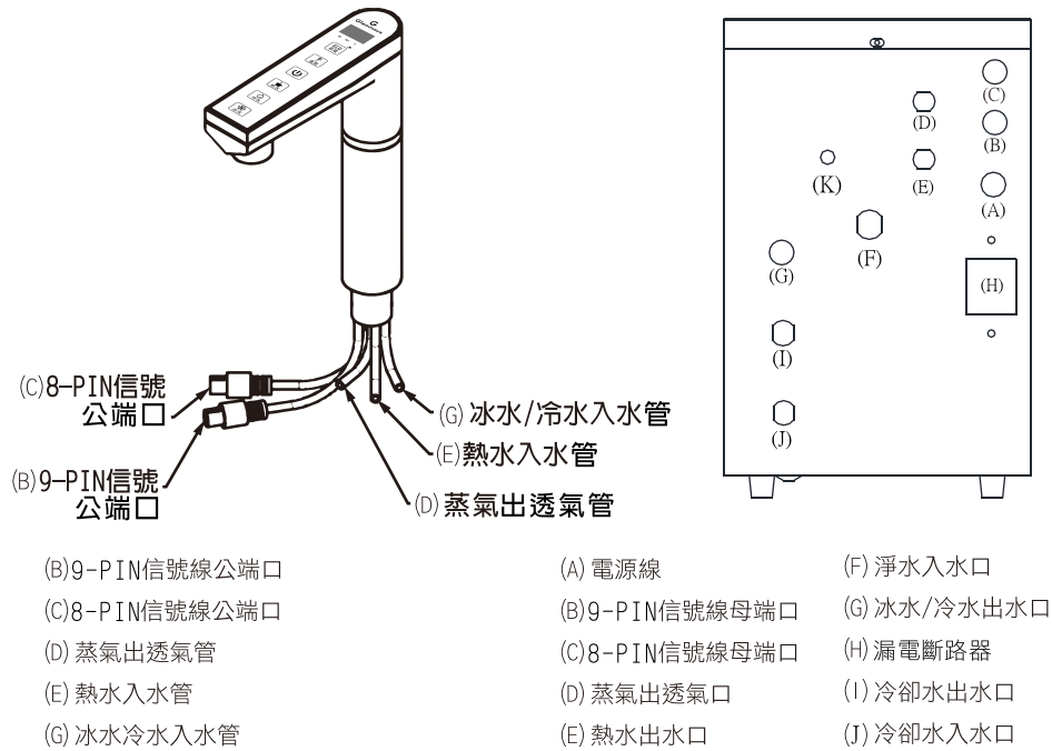
圖B K900
